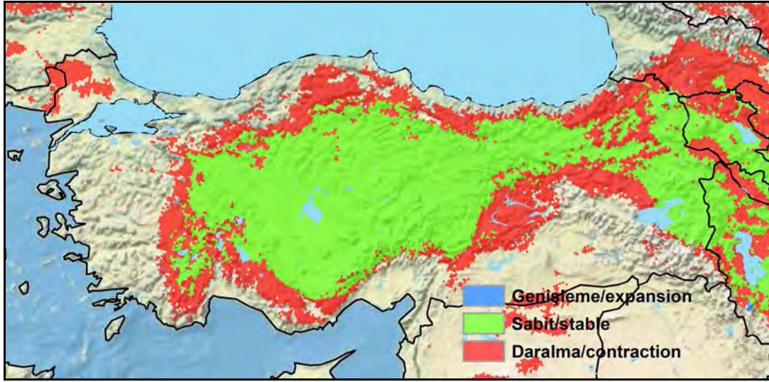
Şekil: Son Buzul Maksimum'dan günümüze Anadolu yer sincabının ( Spermophilus xanthoprymnus ) coğrafi dağılımındaki değişiklikler.
